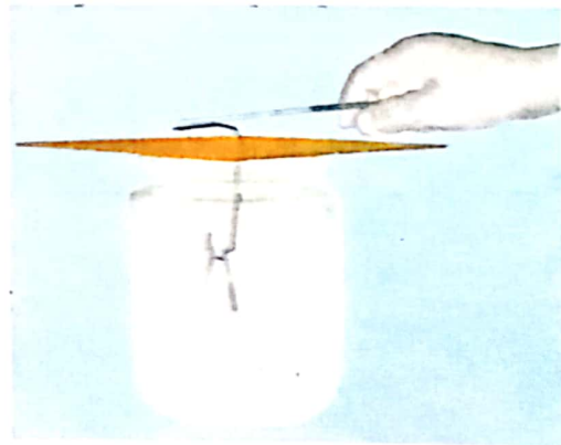
Fig. 13.4 : A Simple Electroscope
