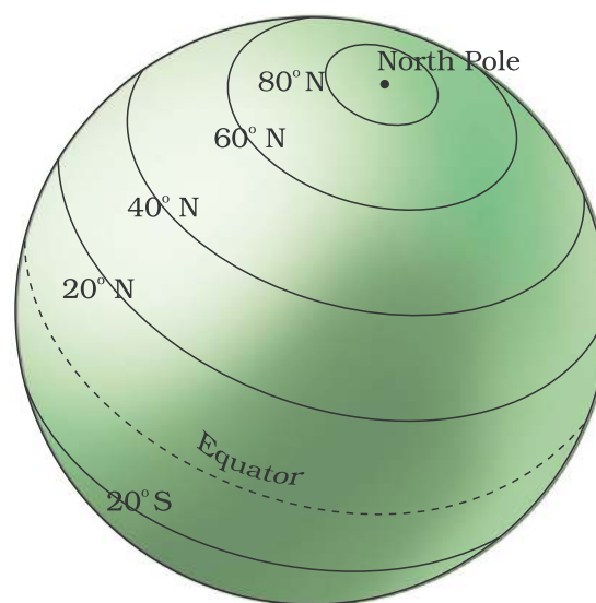
Figure 2.2 : Latitude
